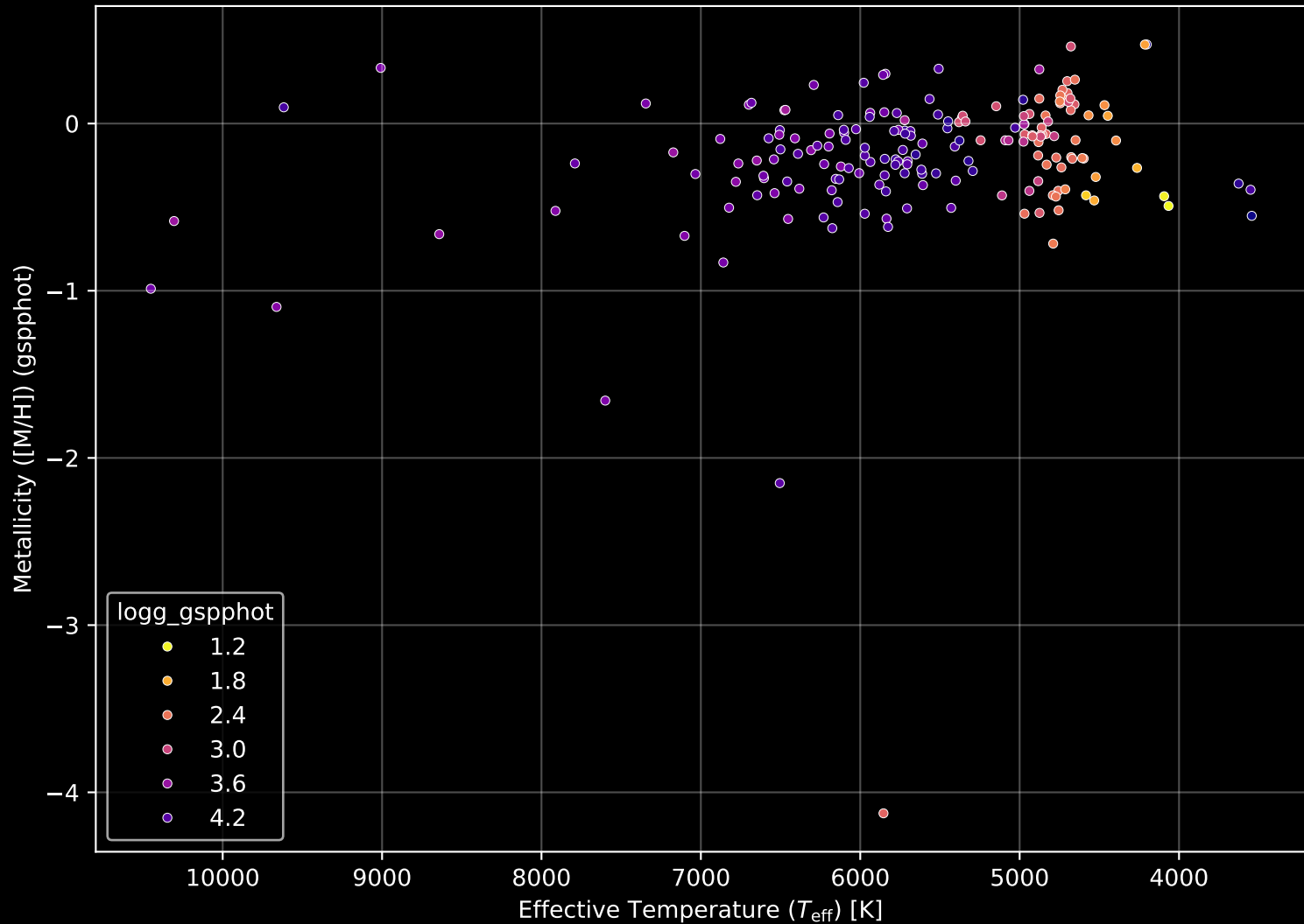
APOGEE DR17 Field: [CVZ_OB15_btx] Stellar Population Parameters (n= 185)
